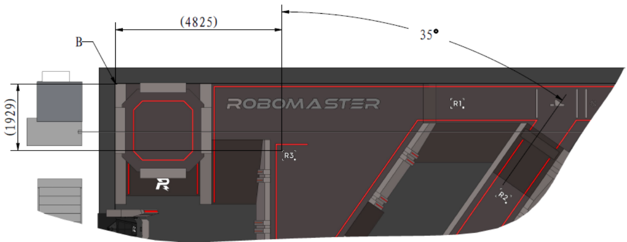
图 2-47 坐标原点和角度示意图
