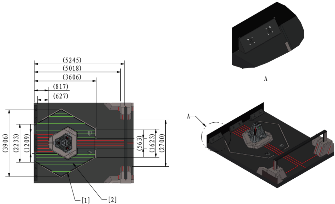
[1] 启动区 [2] 基地增益点
