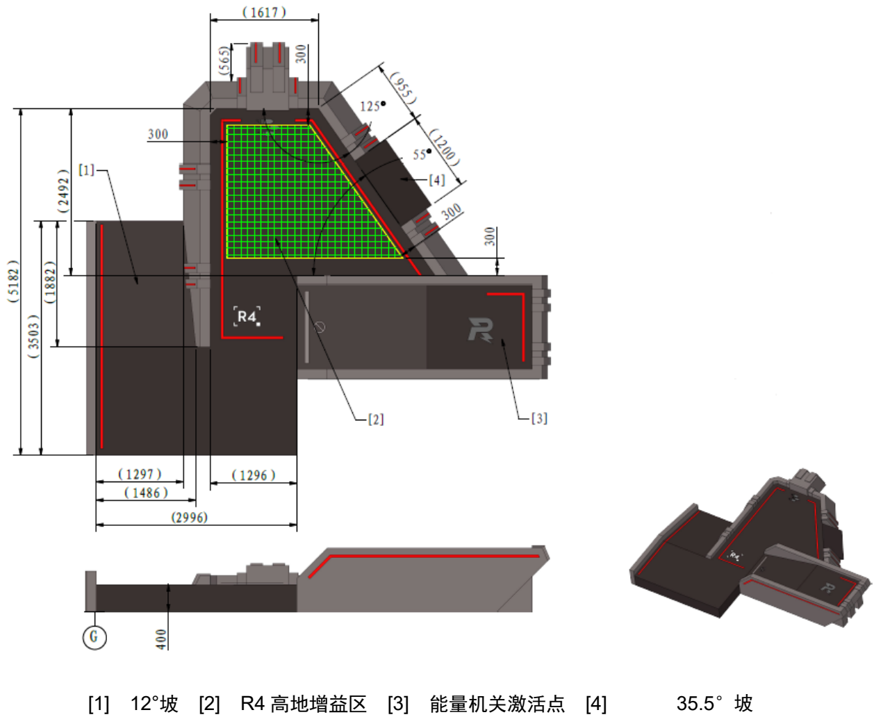
图 2-28 R4 梯形高地示意图
