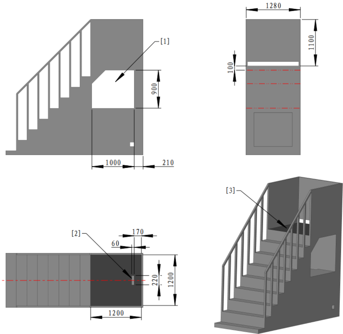
[1] 雷达运算端放置平台 [2] 传感器数据线槽孔 [3] 铁质板材
