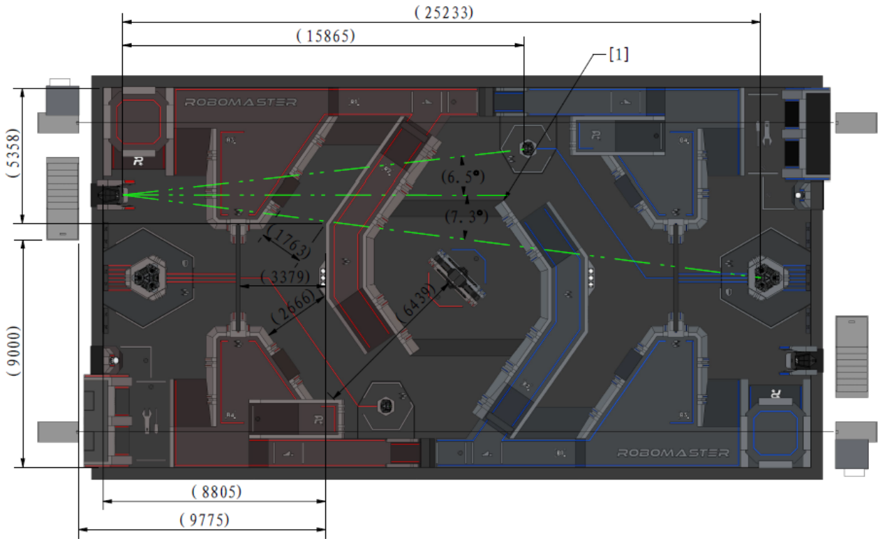
[1] 与战场场边平行且为飞镖发射站朝向
