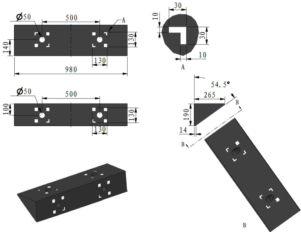
图 2-42 障碍块示意图
