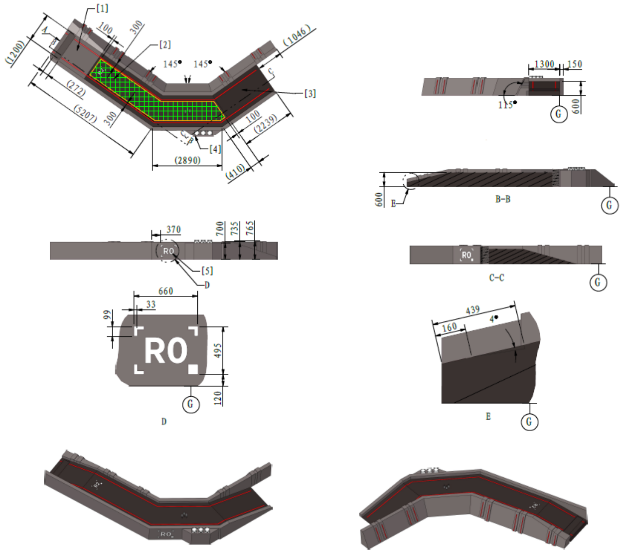
[1] 13°坡 [2] 高地增益点 [3] 15°坡 [4] 小资源岛 [5] 场地定位标签
