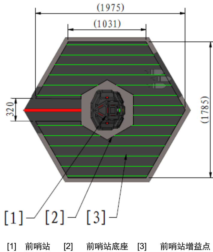
图 2-38 前哨站示意图
