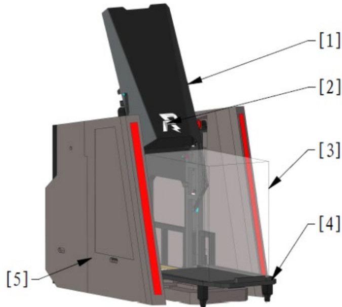
[1] 闸门 [2] 状态指示灯 [3] 飞镖发射架放置空间 [4] 滑台 [5] 发射站主体
